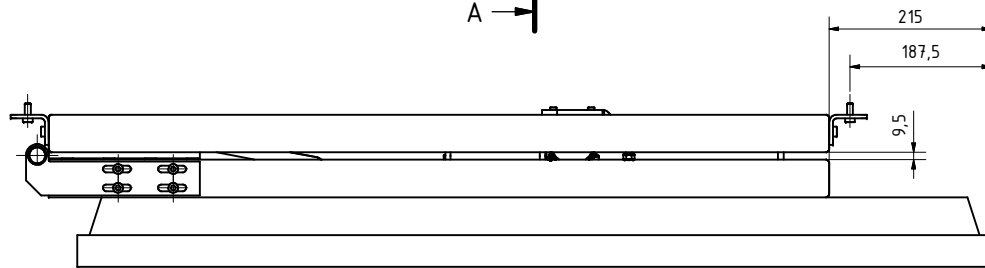
B-B ( 1 : 5 )
