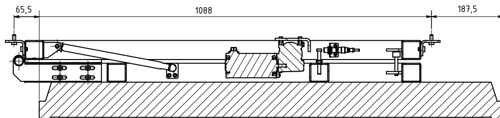
B-B ( 1 : 5 )
