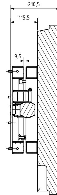
A-A ( 1 : 5 )
